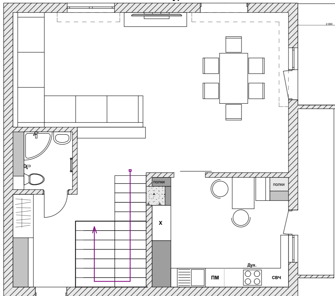
ПЛАН 1 уровень
